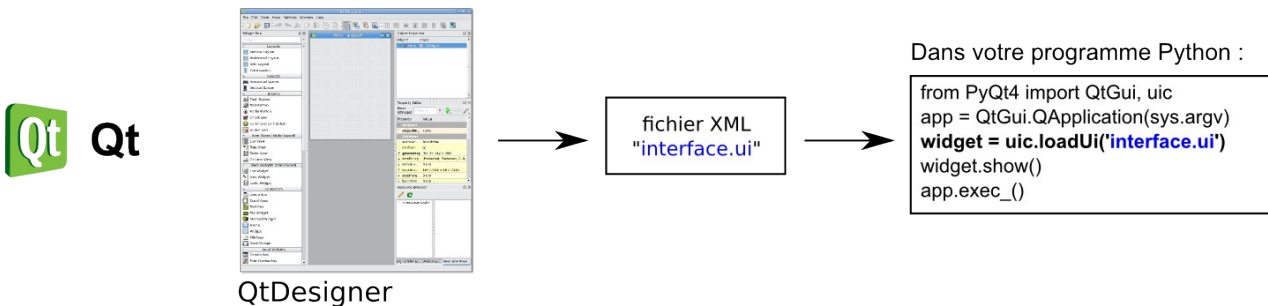
Le logiciel Qt Designer permet de créer visuellement une interface graphique en Qt.
