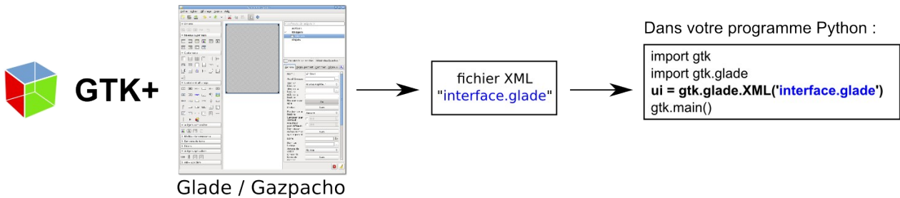
Le logiciel Glade permet de créer visuellement une interface graphique en GTK+.
