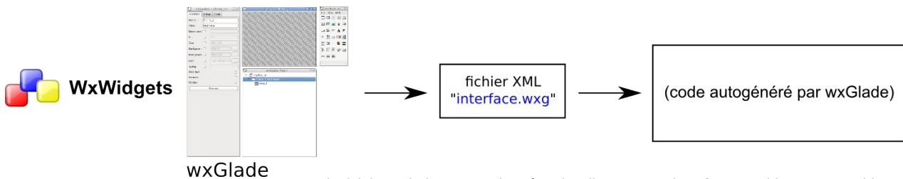
Le logiciel WxGlade permet de créer visuellement une interface graphique en WxWidgets.
